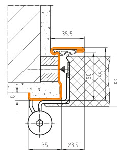
przekrój ościeżnicy
