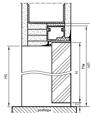
Przekrój pionowy dla drzwi Sara Eco 2 bezprzylgowe
